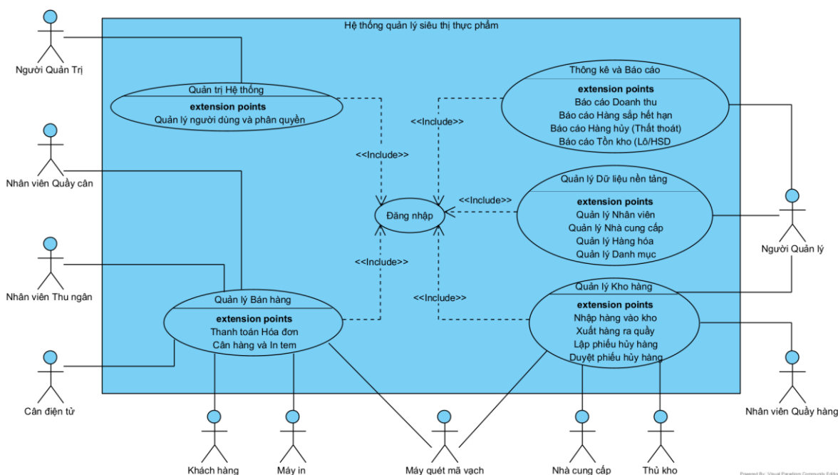
Hình 1. Biểu đồ Use Case Tổng quát
