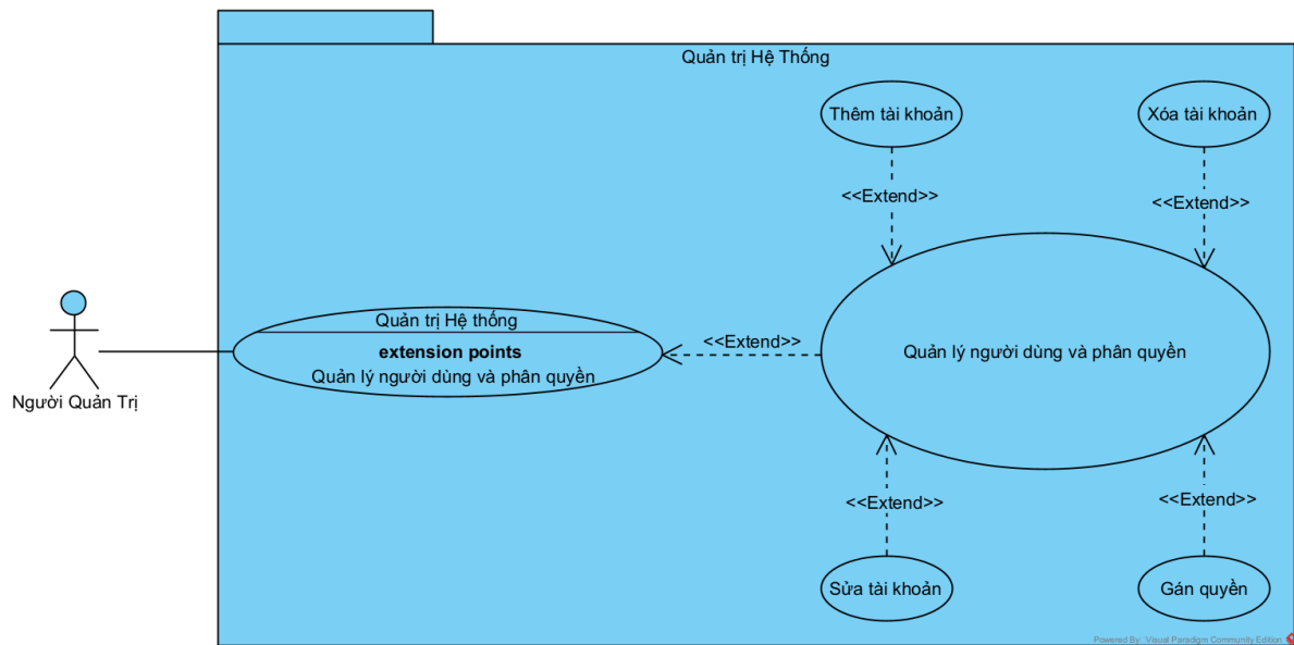
Hình 2. Biểu đồ UC gói Quản trị hệ thống
