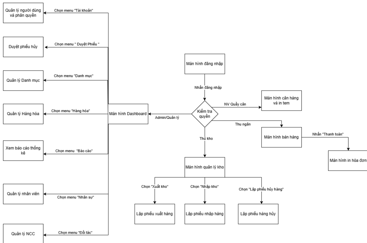
Hình 7. Sơ đồ luồng màn hình
