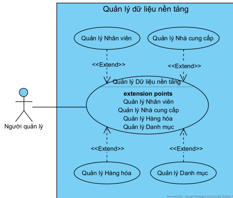
Hình 4. Biểu đồ UC gói Quản lý Dữ liệu nền tảng
