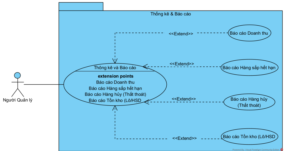
Hình 6. Biểu đồ UC gói Thống kê và Báo cáo
