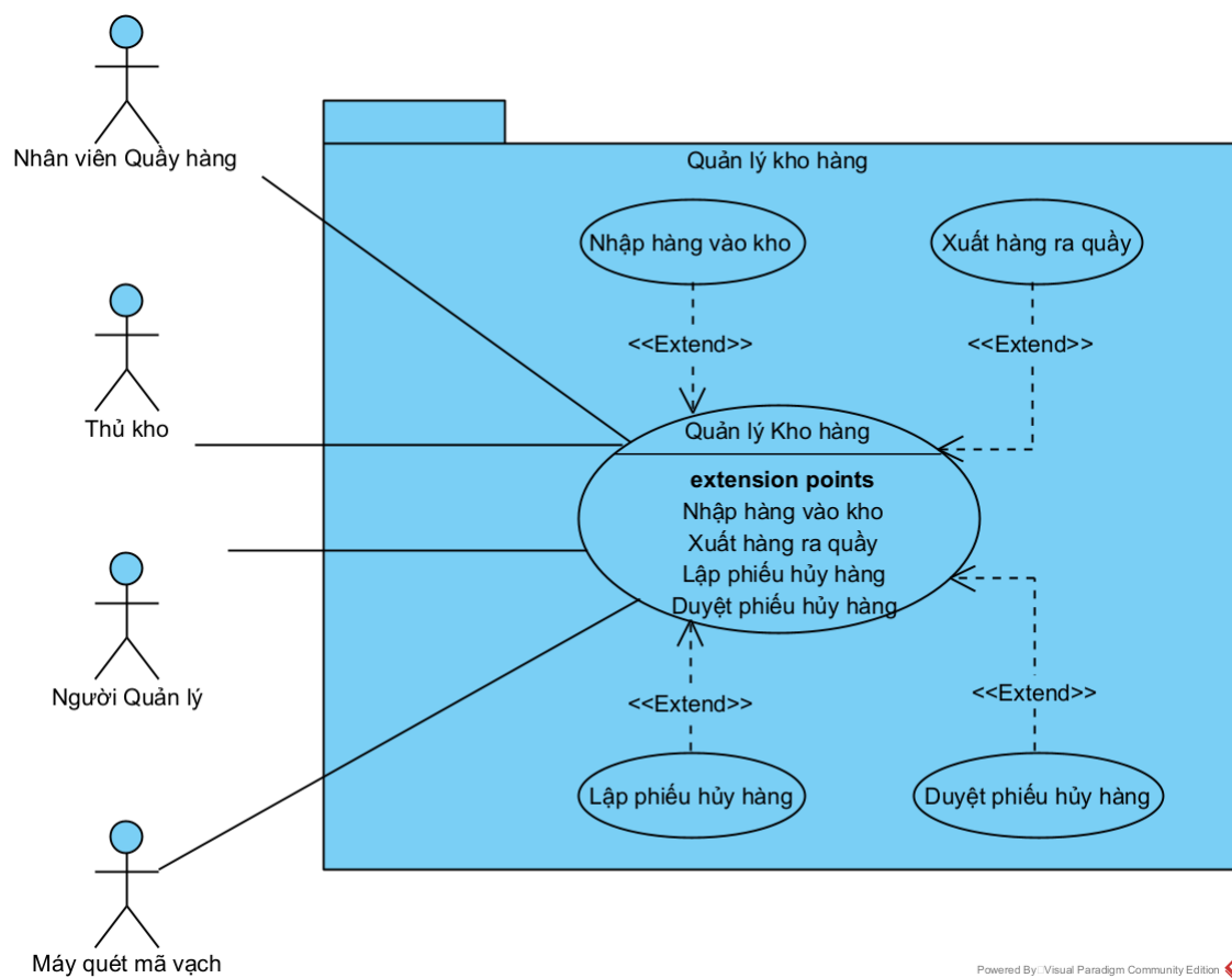
Hình 5. Biểu đồ UC gói Quản lý kho hàng
