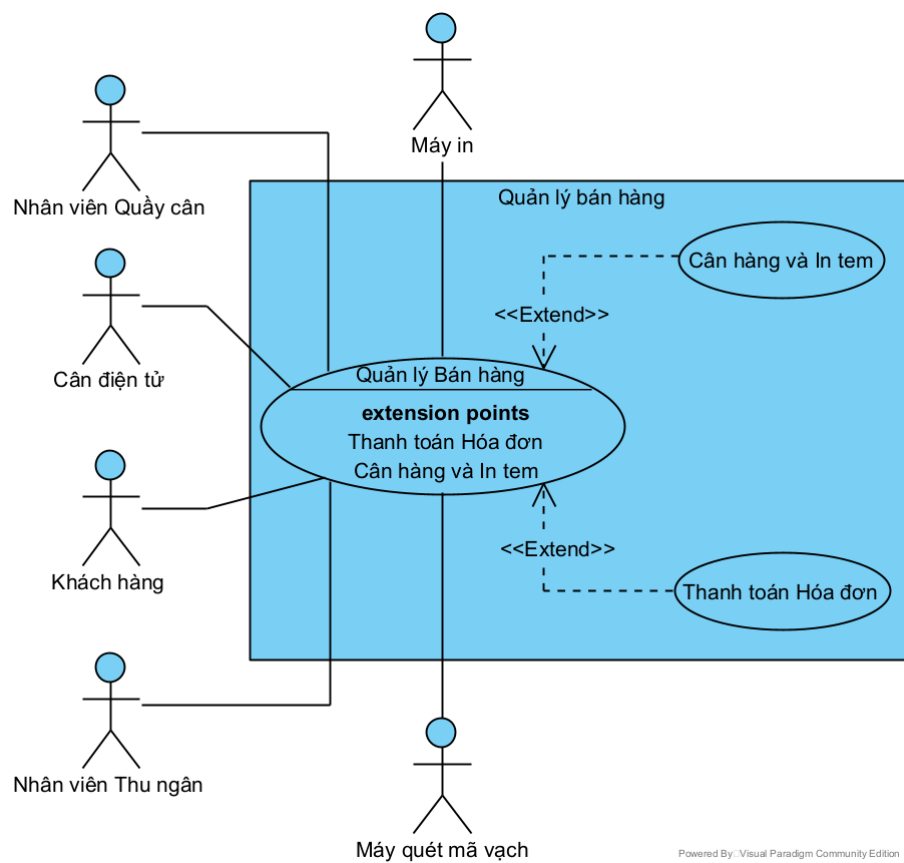
Hình 3. Biểu đồ UC gói Quản lý Bán hàng
